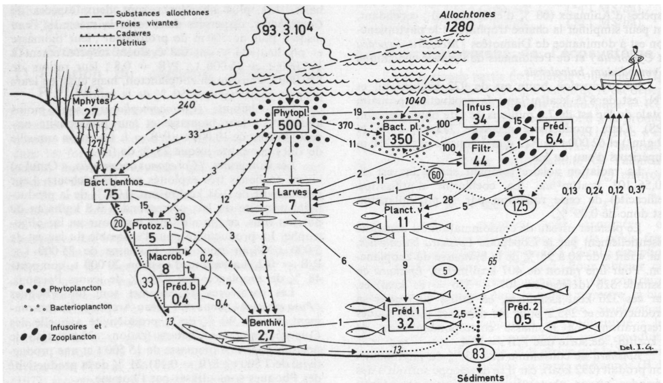
Fig. 4.38 Productivité biologique et flux d'énergie dans l'écosystème « lac-réservoir » à Rybinsk (U.R.S.S.), de 1964 à 1967 (d'après Sorokine, 1972).
