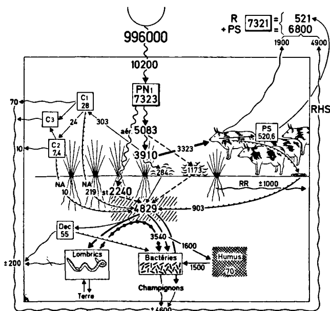
Fig. 4.58 Flux d'énergie (en kcal/m 2 /an) dans une prairie de Normandie (Haras au Pin) (d'après Ricou, 1978). Ondulé court : énergie solaire ; ondulé long : énergie respiratoire (infra-rouge long) ; tireté : matière végétale morte livrée aux décomposeurs ; lignes ponctuées : matières animales mortes livrées aux décomposeurs. RR : respiration des racines ; RHS : respiration des hétérotrophes du sol.
