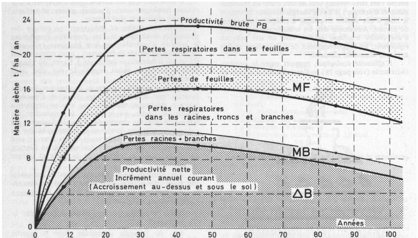
Fig. 4.25 Production (bilan) de la matière sèche d'une hêtraie danoise ( Fagus sylvatica ) de 2 e classe de productivité.
