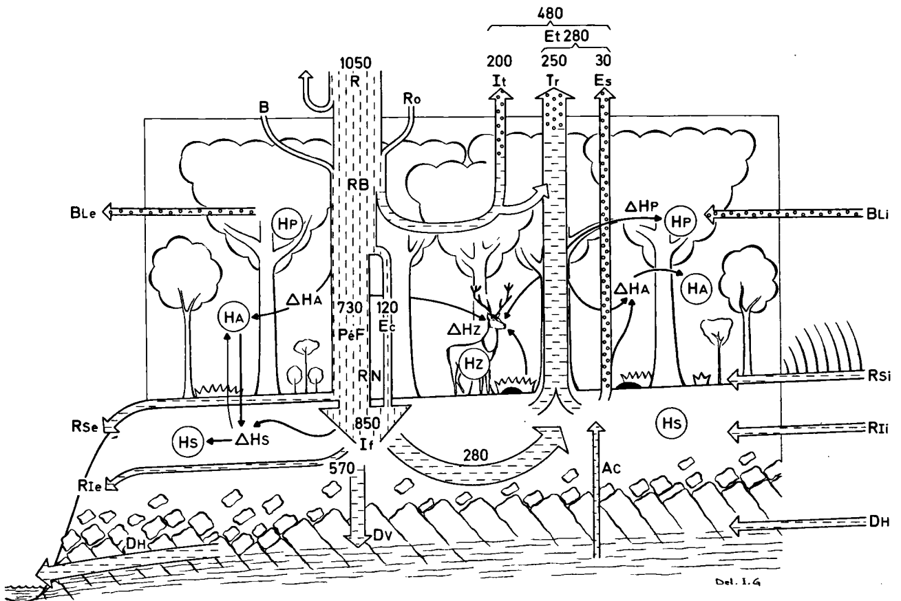
Fig. 4.7 Bilan d'eau dans une biogéocénose forestière. Les chiffres sont ceux de la Hêtraie médioeuropéenne de Mirwart (Belgique) et Solling (R.F.A.). (Pour explications, voir texte.)
