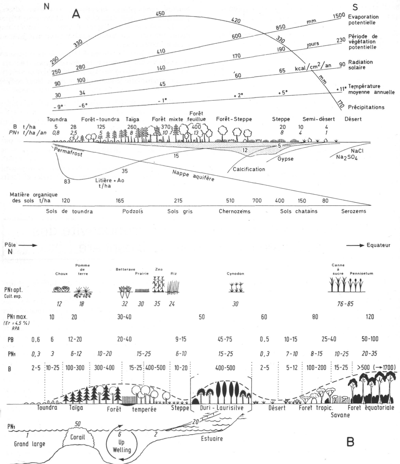
Fig. 4.63 Succession Nord-Sud des principaux zonobiomes et de leurs biomasses et productivités (en t/ha et t/ha/an). A. En U.R.S.S., depuis la toundra jusqu'au désert (d'après Vysotsky, Pogrebnyak et Walter, modifié). B. Du pôle à l'équateur (d'après Rodin, Bazilevitch, Nitchiporovitch, Duvigneaud, etc...). Productivités maximales pour une efficacité de 4,5 % des RPA. Productivités optimales obtenues dans des cultures expérimentales dans des conditions optimales. (Pour explications, voir texte.)
