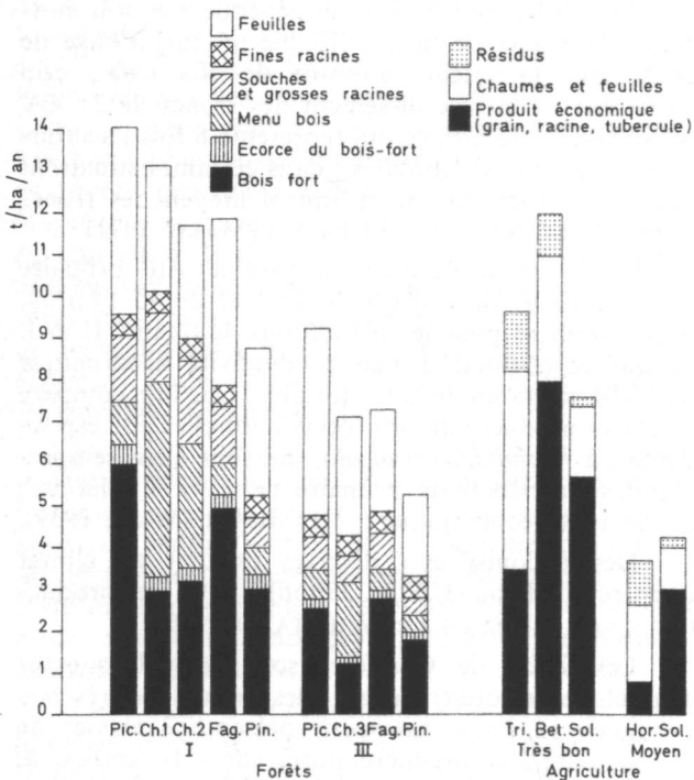
Fig. 4.50 Productivité primaire nette comparée de différents types de peuplements forestiers et de quelques grandes cultures agricoles (d'après Ehwald, 1957 et Duvigneaud, 1971). I et III, classes de bonité en Allemagne, pour Fagus , Picea et Pinus . Chênaies (Ch) de Belgique.
