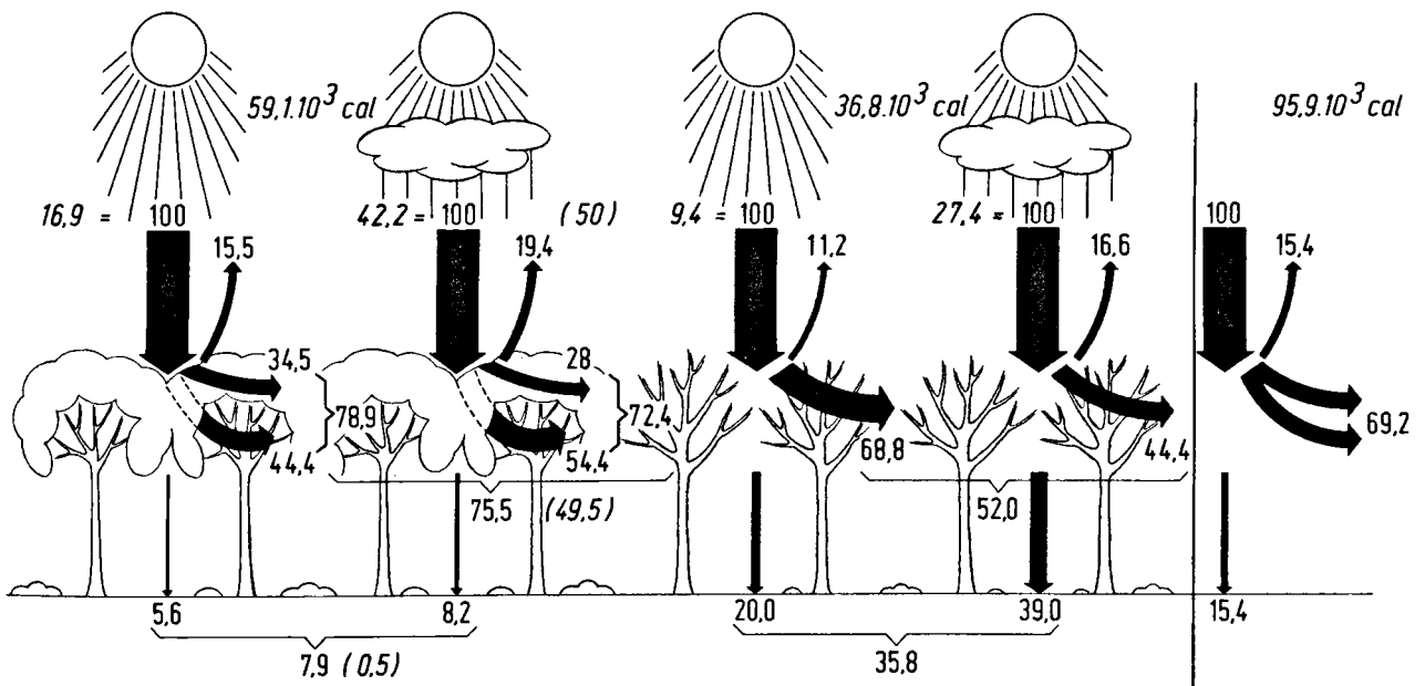
Fig. 4.6 Distribution annuelle de l'énergie (en 10 3 cal/m 2 ) dans une forêt caducifoliée de Belgique (Querceto-Carpinetum à Virelles). Réflexion, interception, transmission, pendant la phase feuillée (ciel clair et ciel couvert), pendant la phase défeuillée (ciel clair et ciel couvert) et pour l'année entière.
