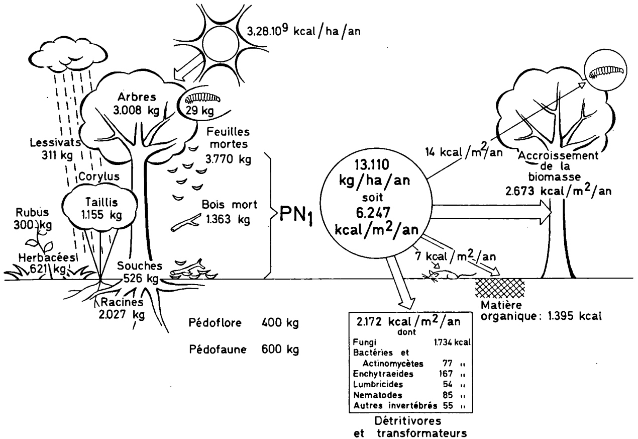
Fig. 4.30 Productivité primaire nette et son utilisation (incrément, productivité secondaire) dans une Chênaie à Corylus de Grande-Bretagne (d'après Satchell, 1971).
