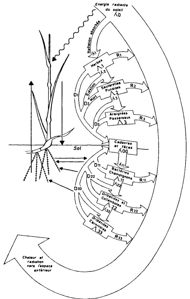
Fig. 4.2 L'écosystème terrestre en tant que superposition de deux systèmes distincts, l'un aérien, l'autre souterrain. Prairie à Poa compressa , dans un « Oldfield » du Michigan, (d'après Engelmann, 1961, modifié). (Pour explications, voir texte.)
