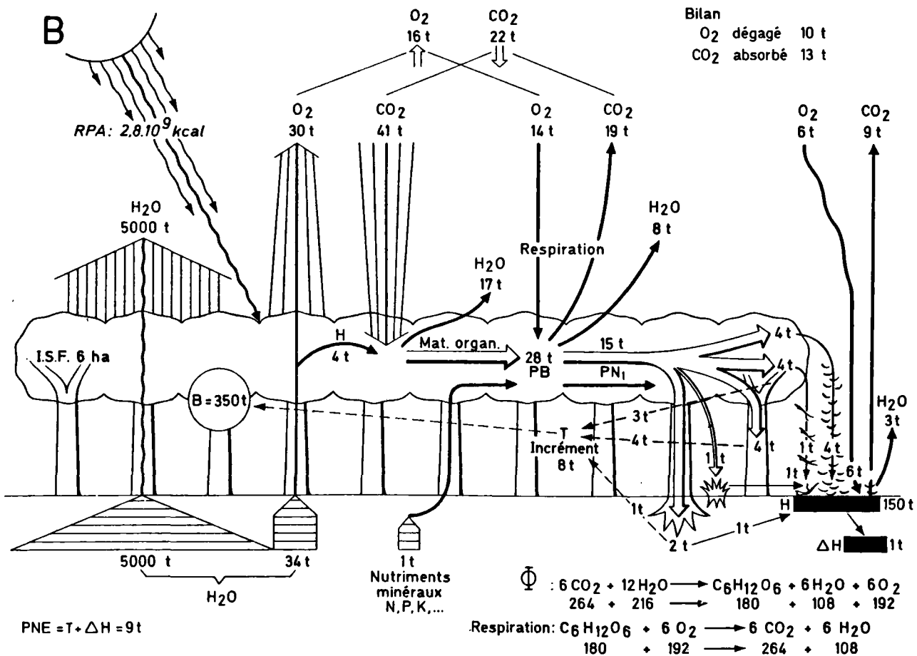
Fig. 4.59 Comparaison du fonctionnement de l'écosystème « Champ de blé » (A) (d'après Ničiporovič, modifié) avec celui de l'écosystème forêt caducifoliée (B). Valeurs à l'ha. (Pour explication, voir texte.)
